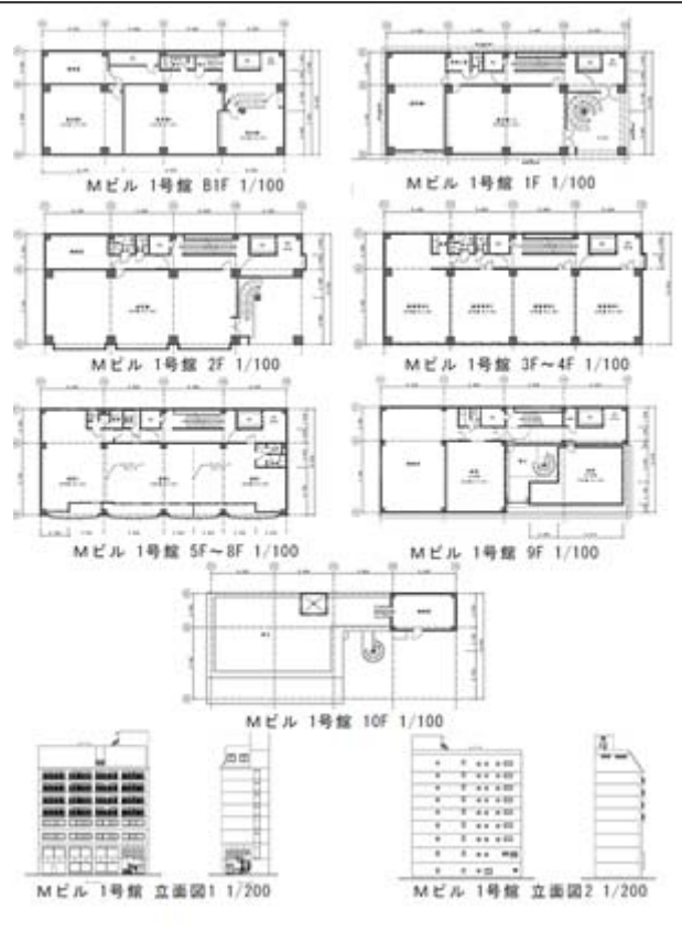
Mビル1号館平面図拡大する
