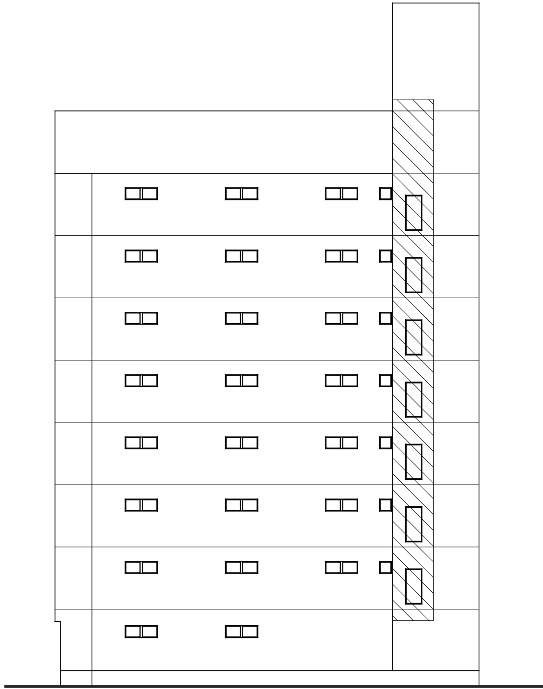
北立面図
