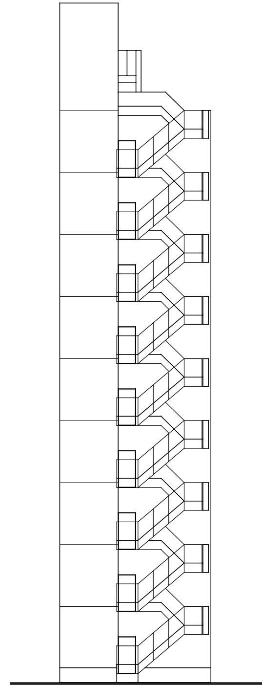
西立面図
