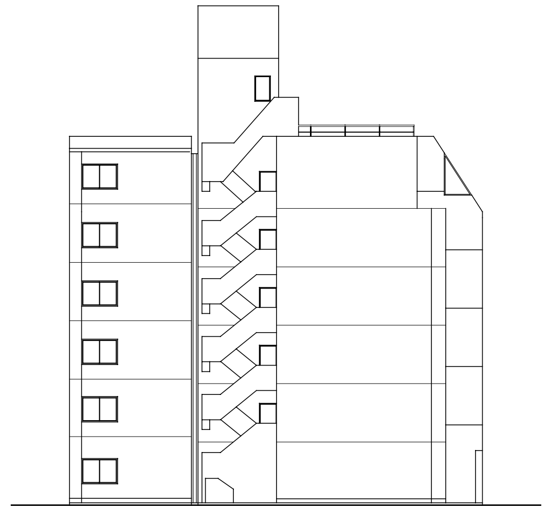
南立面図
