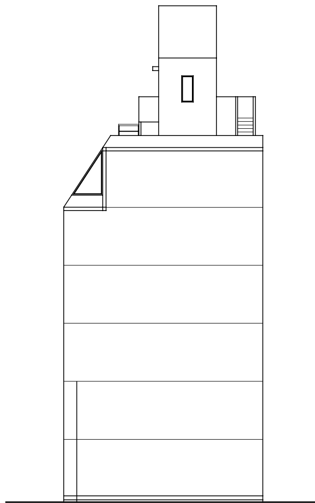
西立面図
