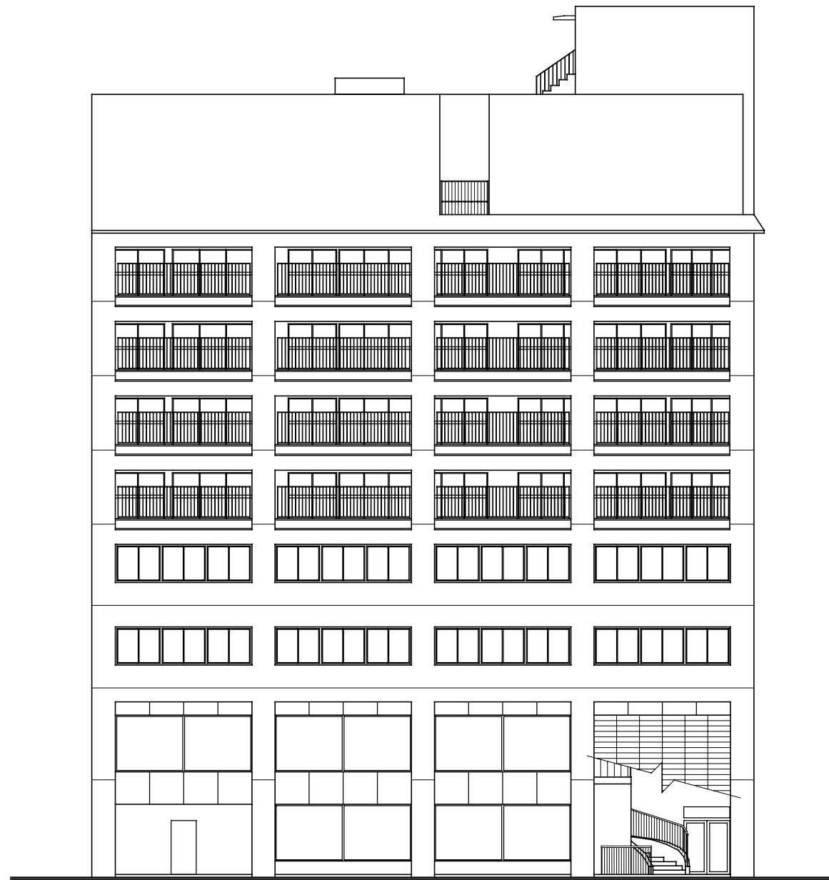
南立面図
